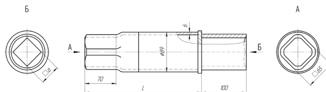
Штанга стационарная типа ШС
